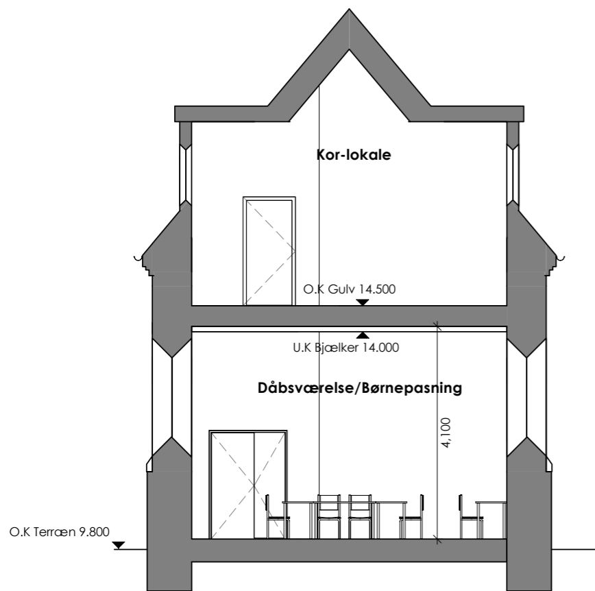
Snit B-B
