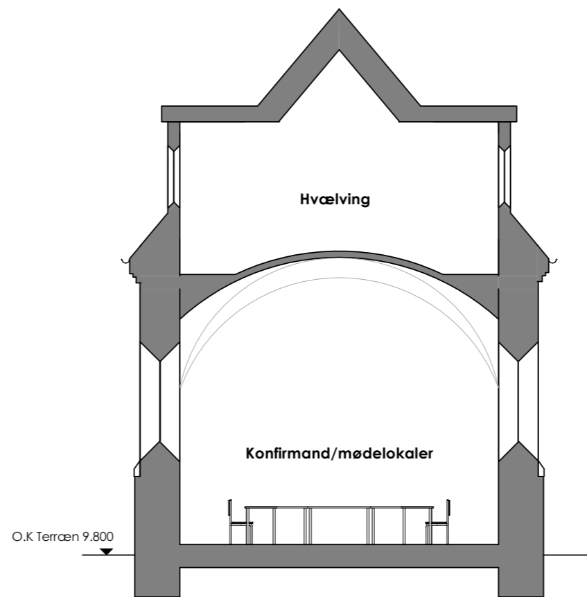
Snit C-C
